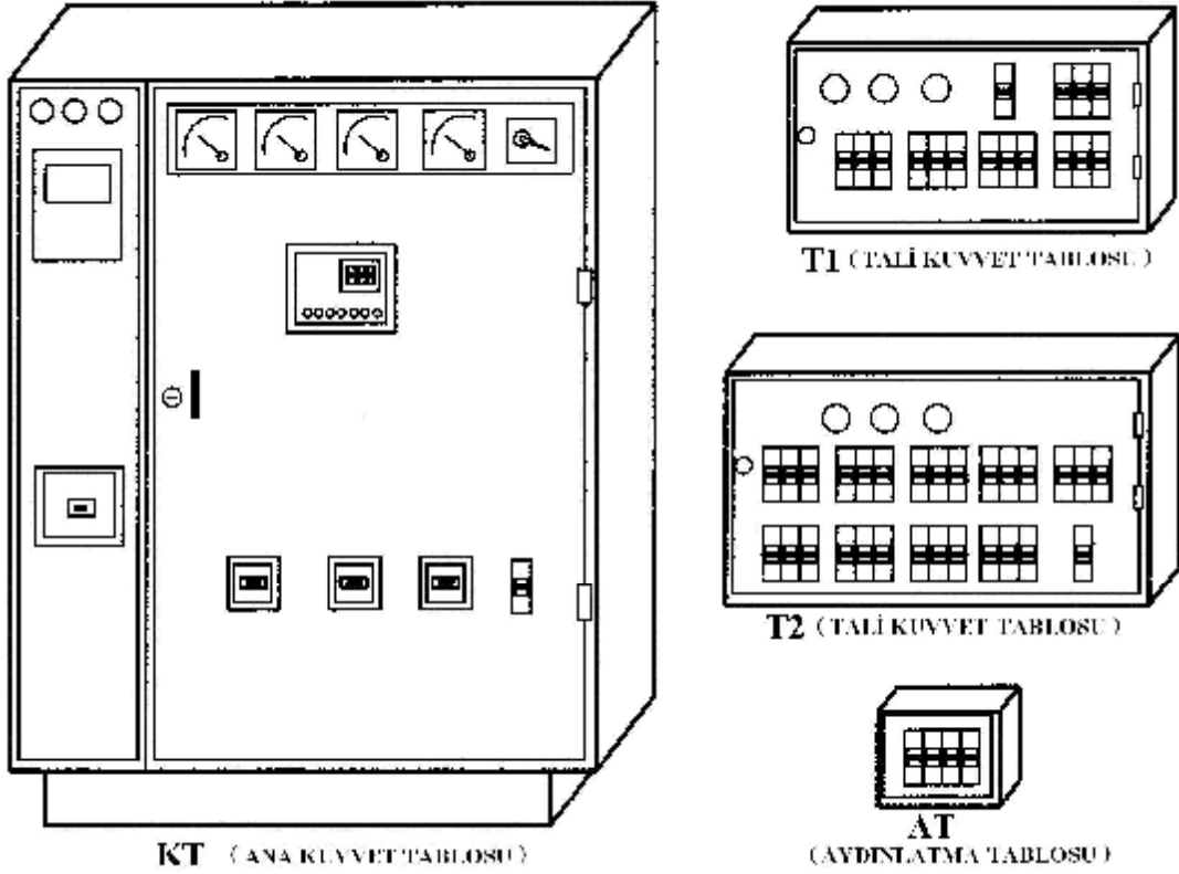
Şekil 3.3: Tablo çizimleri
