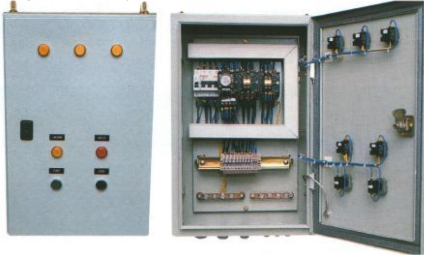
Resim 3.4: Kumanda tablosu
