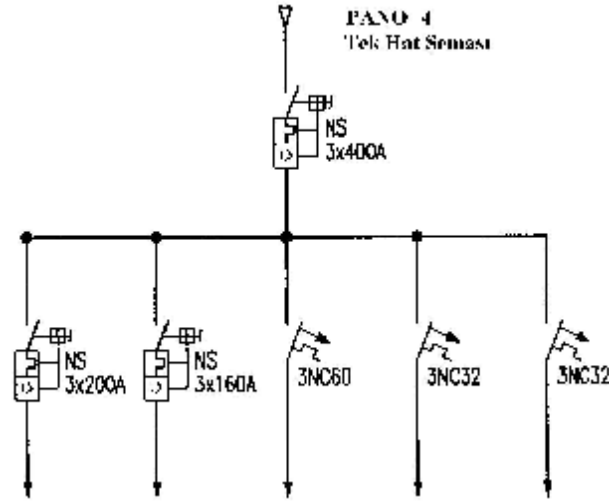
Şekil 3.16: Ana dağıtım tablosundan beslenen 4 nolu panoya ait kolon seması
