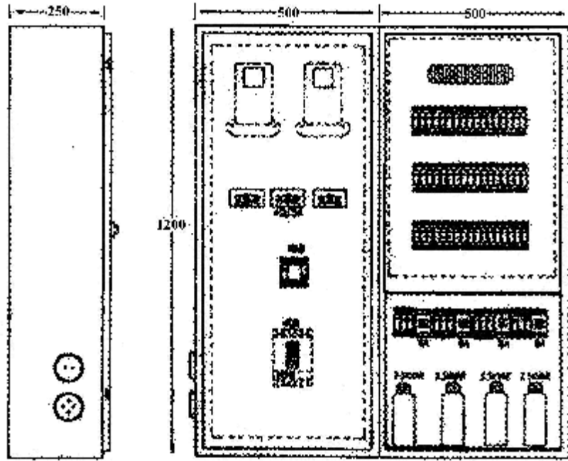
Şekil 3.7: Kompanzasyon panosu (Kapakların açık hali)
