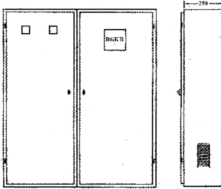
Şekil 3.6: Kompanzasyon panosu (Kapakların kapalı hali)
