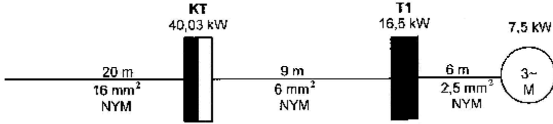
Şekil 1.4: Gerilim düşümü hesabı
